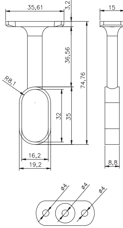
Kapaalı Oval Boru Babası
