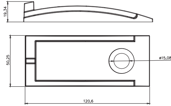
Dökdörtgen Kapı Takteği
