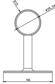
Kapalı Boru Babası
