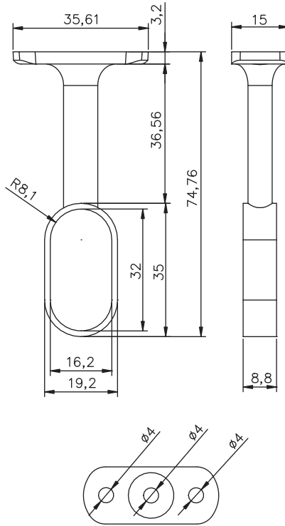
Açık Oval Boru Babası
